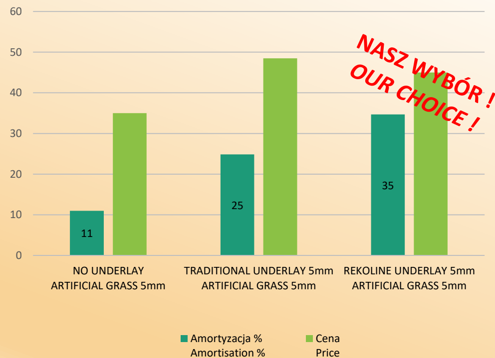
UKŁAD ZE SZTUCZNĄ TRAWĄ SYSTEM WITH ARTIFICIAL GRASS
