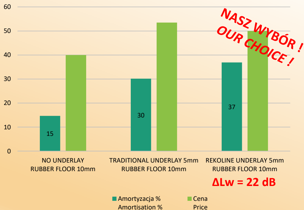
UKŁAD Z MATĄ GUMOWĄ 10mm SYSTEM WITH RUBBER MAT 10mm
